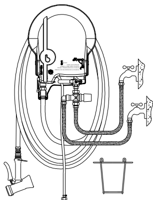
MITIGEUR THERMOSTATIQUE PMITI00002
